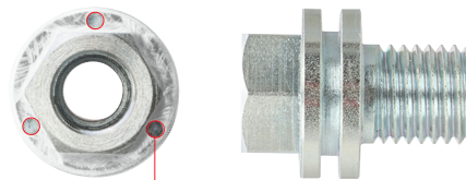
ワイヤロック穴 φ2.0 / 3箇所
